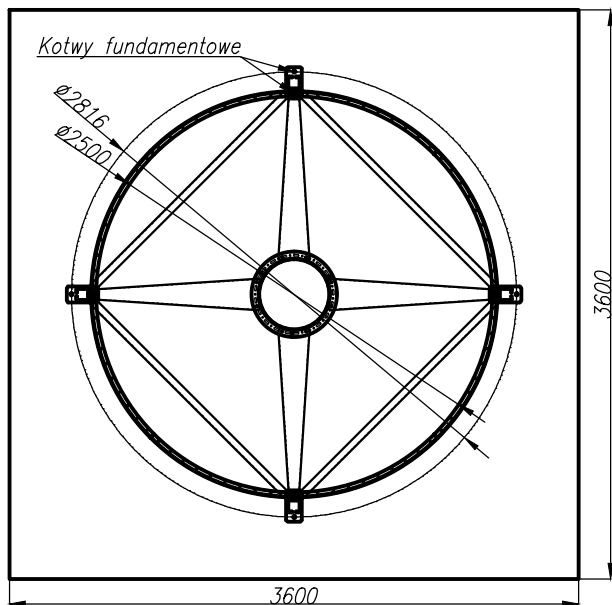
Posadowienie na płycie fundamentowej.
