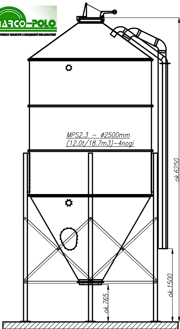
Posadowienie na płycie fundamentowej.
